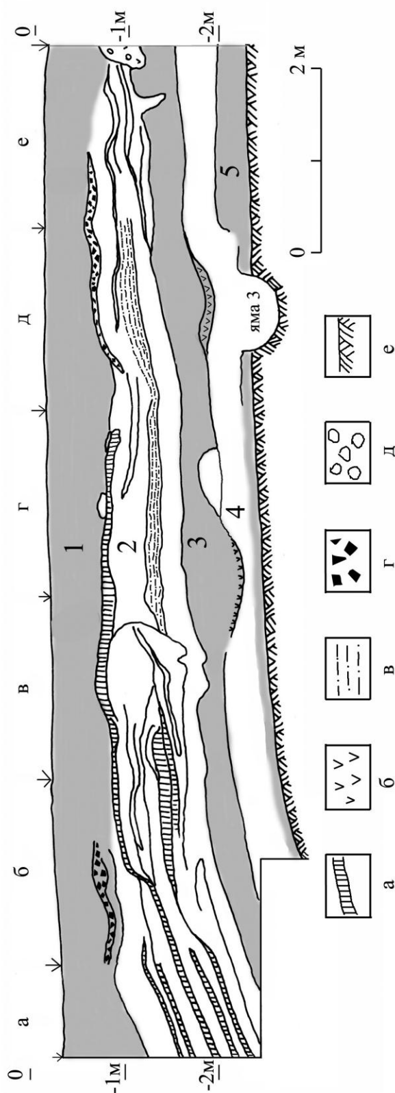
Рис. 6. Стратиграфічний профіль західної стінки розкопу в Дубні по вул. Замковій, 10. Умовні позначення: а – шар суглинку; б – вугілля і попіл; в – шар органічного ґліну; г – бита цегла; д – шматки печини; е – материк.
