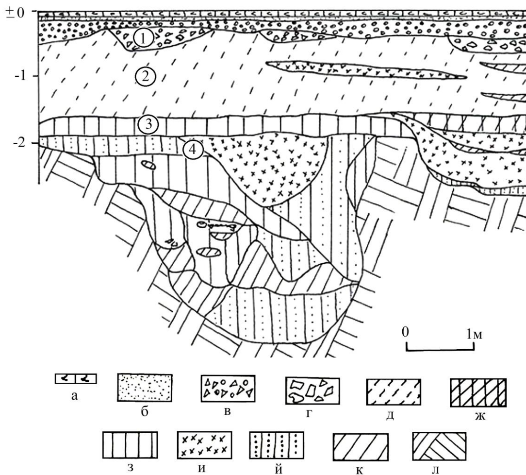
Рис. 14. Стратиграфічний профіль південно-східної стінки (з перерізом споруди № 2) розкопу в Корці по вул. Київській, 61-б. Умовні позначення: а – бруківка; б – пісок; в, г – дрібні та великі шматки будівельного сміття; д – шар сірого ґрунту; ж – пласт суміші глини та ґрунту; з – шар чорного ґрунту; и – скупчення органіки; й – шар чорного ґрунту із вкрапленнями вапна; к – глина; л – материковий суглинок. 1 – ґрунт з будівельним сміттям ХІХ–ХХ ст.; 2 – шар сірого кольору насичений матеріалами ХVІІІ–ХІХ ст.; 3 – культурний шар ХVІІ–ХVІІІ ст. чорного кольору; 4 – заповнення споруди № 2 кінця ХVІ – першої половини ХVІІ ст.
