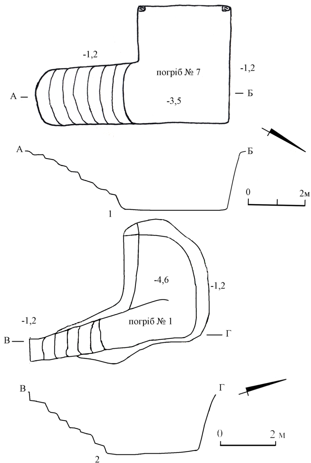
Рис. 50. Плани та розрізи погребів кінця XVI – першої половини XVII ст.: 1 – Дубно; 2 – Острог.
