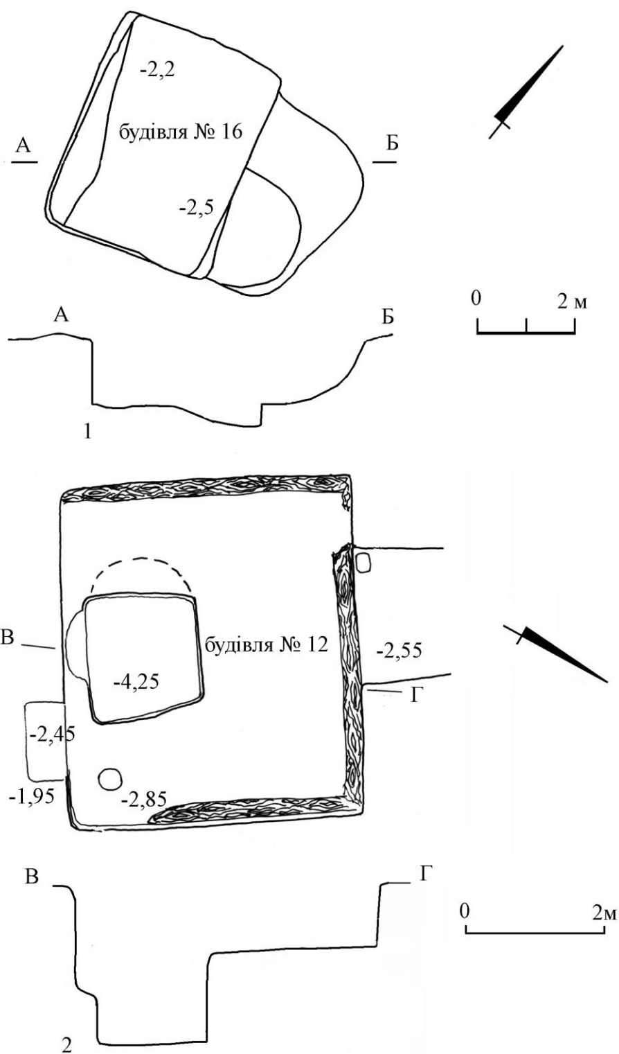
Рис. 46. Плани та розрізи котлованів житлових будівель XV–XVI ст.:
