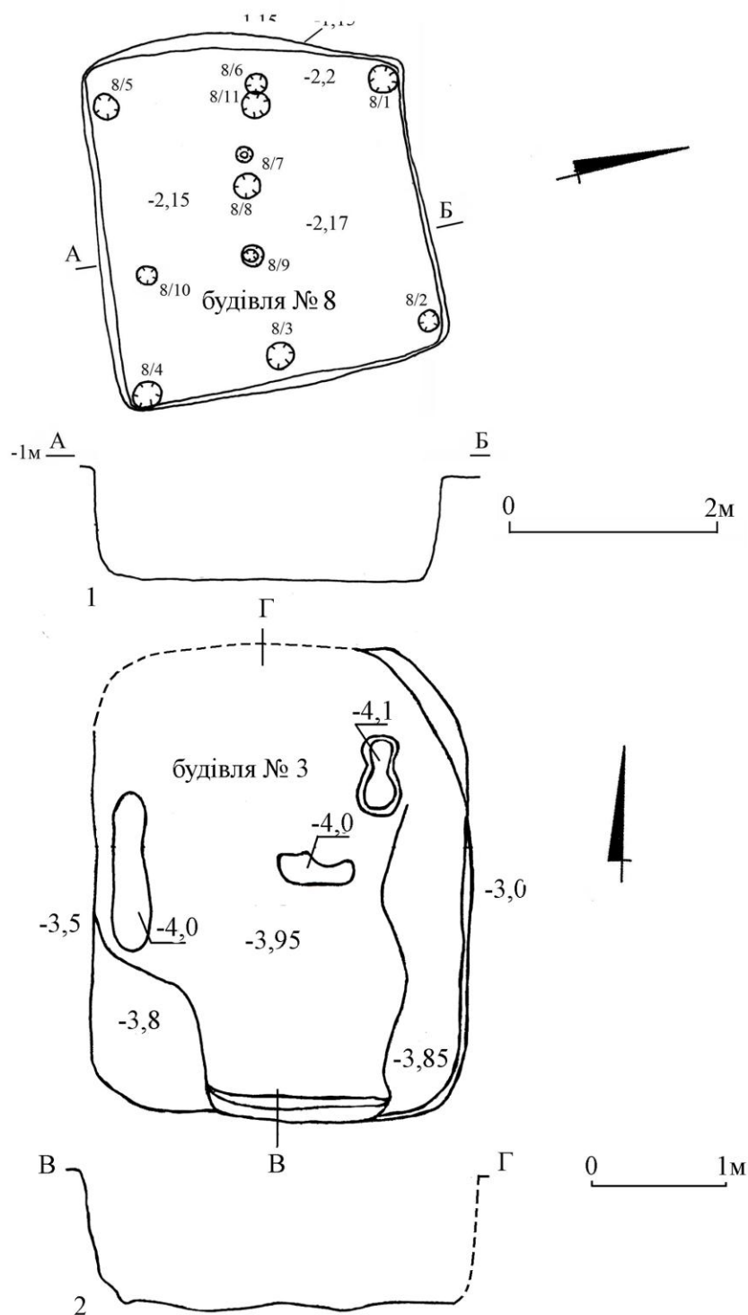
Рис. 45. Плани та розрізи котлованів житлових будівель XV–XVI ст.:
