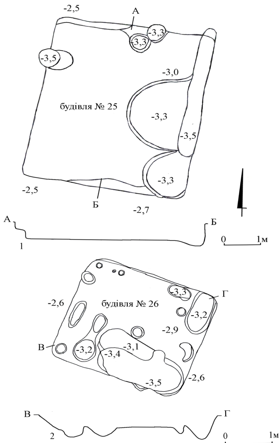
Рис. 48. Плани та розрізи котлованів господарських будівель кінця XVI – першої половини XVII ст.: 1, 2 – Рівне.
