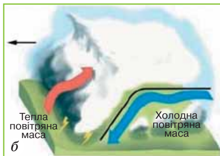
Мал. 63. Атмосферні фронти:
