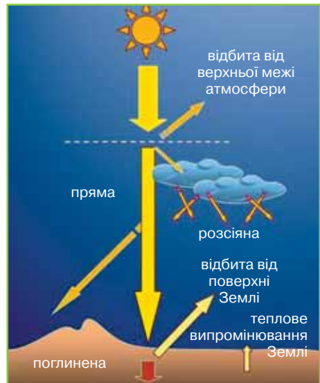
Мал. 62. Види сонячної радіації
