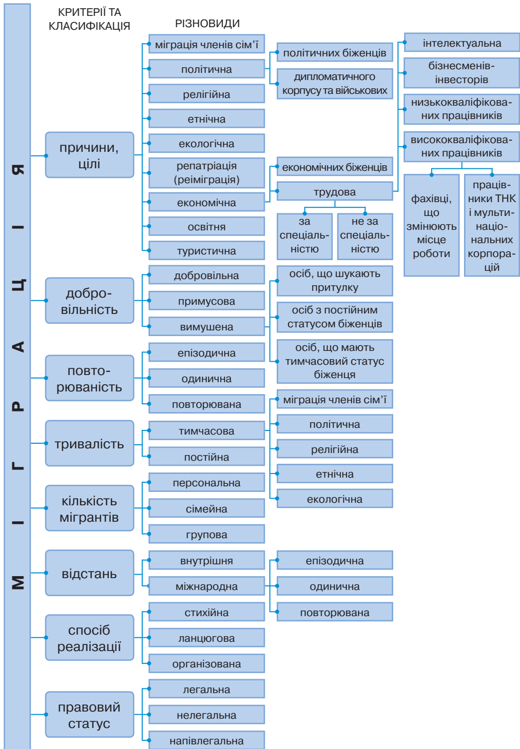
Мал. 154. Класифікація міграцій
